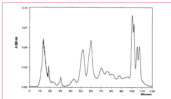
Abbildung 1: Beispiel einer Gliadinauftrennung der Sorte Lux am Kationenaustauscher unter nativen, milden Bedingungen (9 bar Druck, 25°C, 50 mM \text{KH}_2\text{PO}_4 , 2M Urea, pH 3,1)
