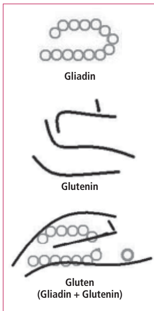
Abbildung 7: Naturwissenschaftliche Modellvorstellung der Kleberanordnung in Weizenmehlen. Glutenine bilden Strang-ähnliche Aggregate, Gliadine dienen als „Gleitmittel“ zwischen den aggregierten Gluteninen
